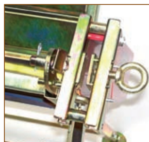
SUPPORTO MOTOSEGHE CON SERRAGGIO A MORSA
